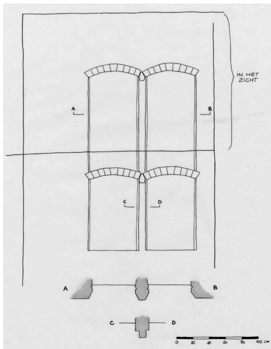
Opmetingsschets met aanzicht en doorsneden van het gemetselde kruisvenster op de verdieping van de oostelijke gevel van het achterhuis van Brugstraat 18. Slechts het bovenste deel was zichtbaar; de verticale lijn geeft de dakhoogte van de achterbouw van Brugstraat 16 aan.
