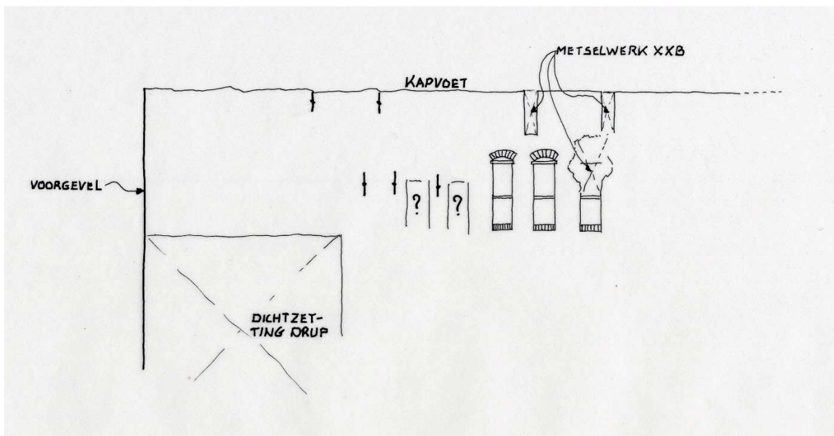
Opmetingstekening van de bouwpozen in de noordgevel. De hoogte van de muur is niet bekend noch de diepte van het voorhuis.
